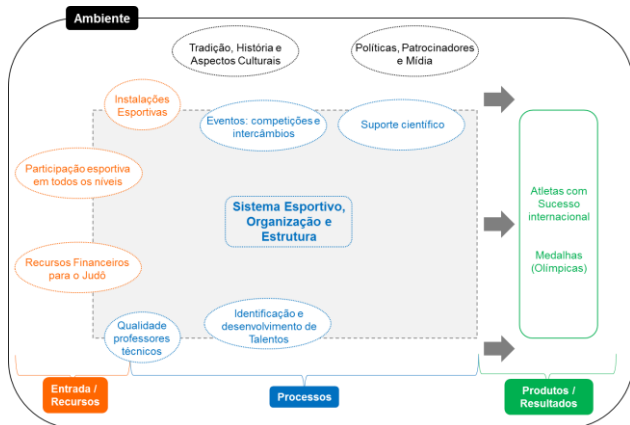
Figura 1. Modelo JUDO-OFIISS.
