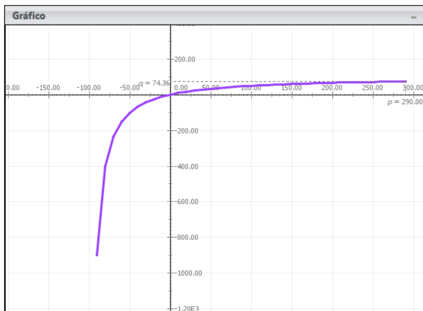
Gráfico 2 – Distância do objeto em relação a distância da imagem para um espelho convexo
