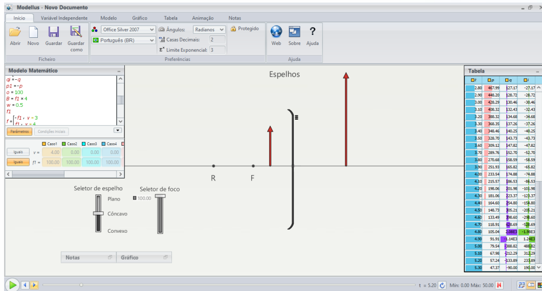
Figura 6 – Representação do objeto entre o foco e o vértice de um espelho côncavo. Fonte: próprio autor
