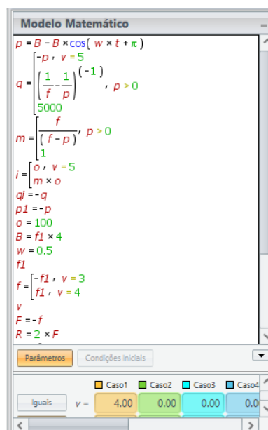
Figura 2 – Janela da modelagem matemática para simulação no software Fonte: próprio autor
