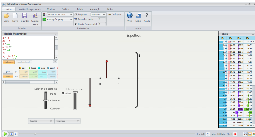
Figura 5 – Representação do objeto entre o centro de curvatura e o foco de um espelho côncavo Fonte: próprio autor
