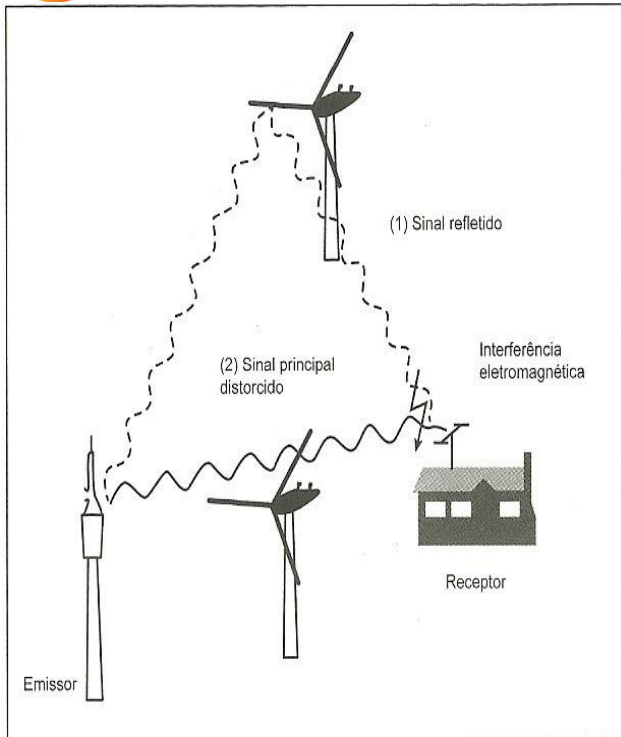
Figura 4 – Espalhamento dos sinais eletromagnéticos.
