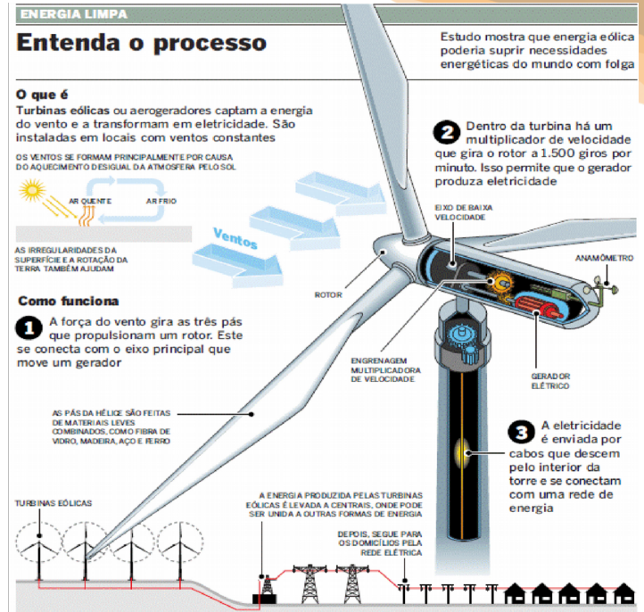
Figura 1 – Aerogerador – Princípio de Funcionamento.
