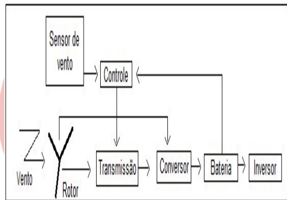
Figura 2 - Diagrama de bloco de um sistema eólico
