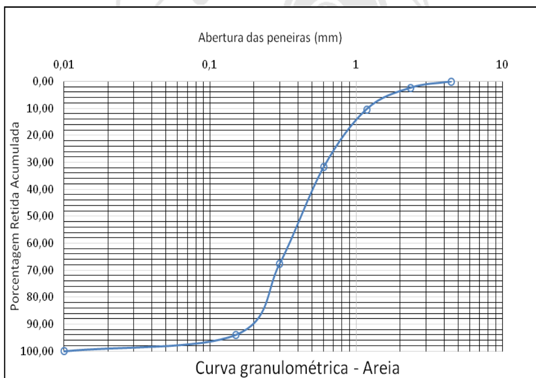
Figura 1: Curva Granulométrica da areia
